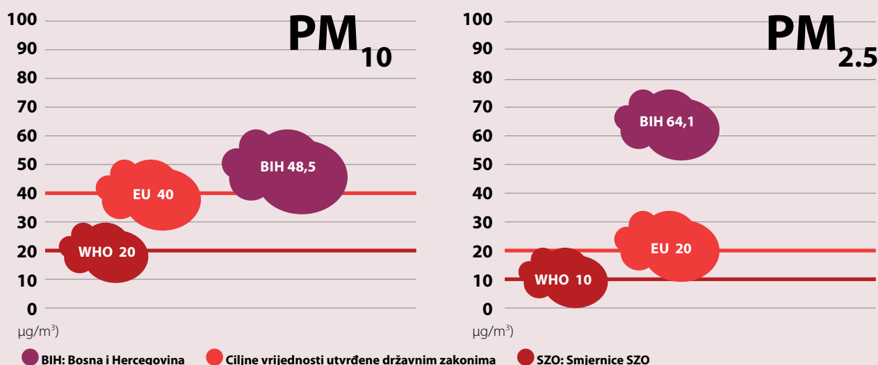
Slika 3. Prosečne godišnje koncentracije PM_{10} i PM_{2.5} u Bosni i Hercegovini i ciljne vrijednosti (koje treba da se postignu do 2021. godine) utvrđene državnim zakonom i smjericama SZO
